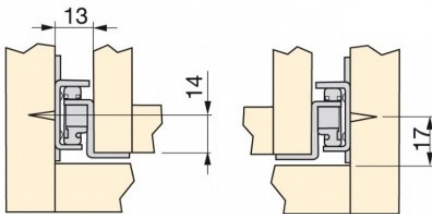
GUIDA A RULLO PER CASSETTI CON FISSAGGIO A SQUADRA E BLOCCO FINE CORSA
