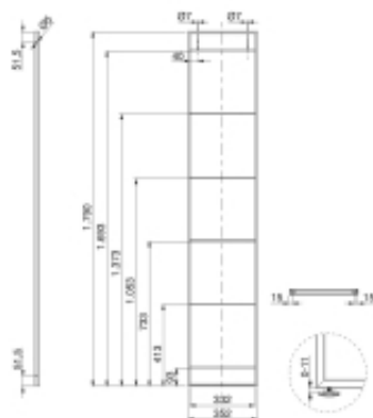
Scaffale Lader. 1790. Verniciato nero, Acciaio
